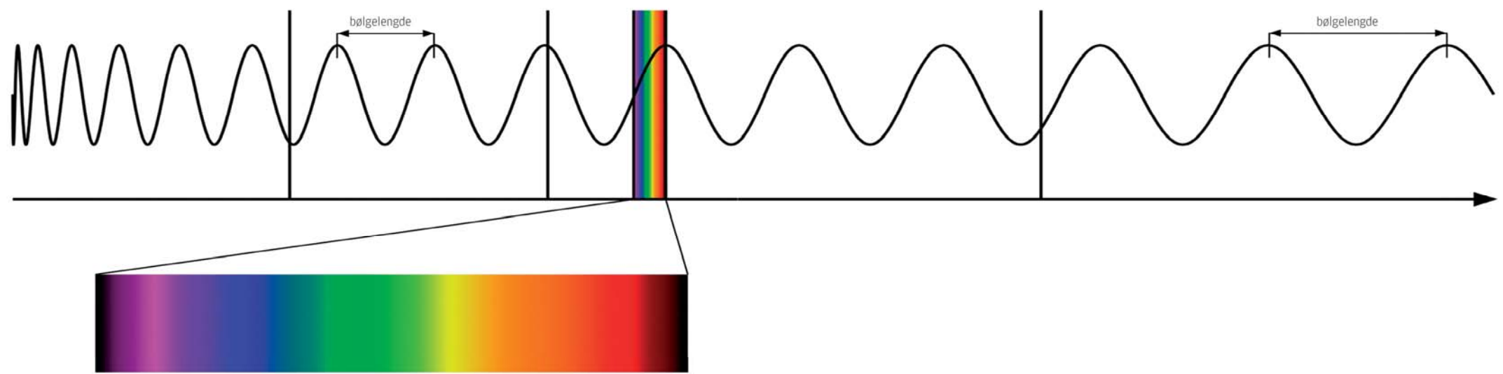
Gammastråling alt under 0,03 nm Røntgenstråling 0,03 nm til 30 nm Ultrafiolett stråling 30 nm til 400 nm Synlig lys 400 nm til 700 nm Infrarød stråling (varmestråling) 700 nm til 14 000 nm Mikrobølgestråling 1 mm til 1000 mm (1m) Radiobølgestråling Over 1 m
